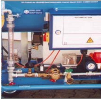
Kompakt-Wasserarmatur mit integriertem Niederdruckminderer.
