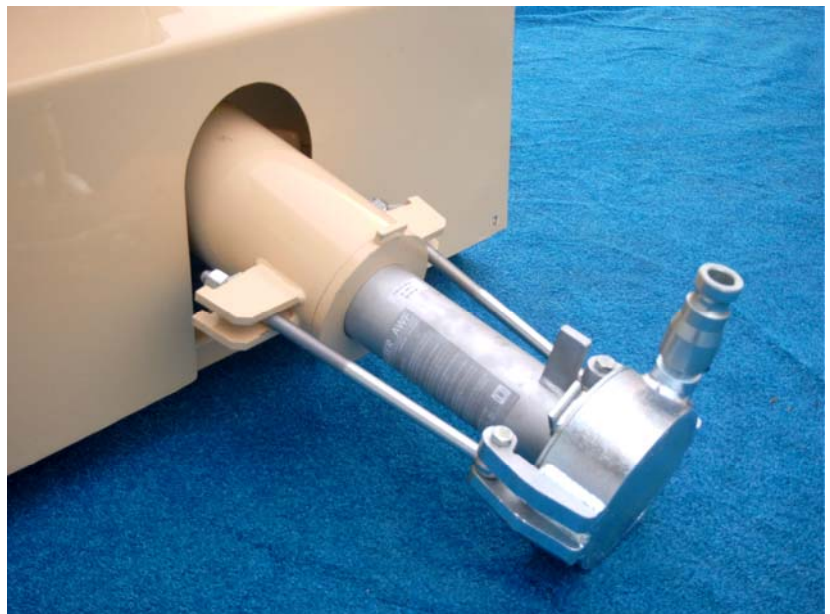
Sicht auf die Schneckenpumpe, hier mit montiertem Nachmischer mit Pumpenabgang
